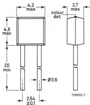
Fig.1 Type 2322 640 90004.
