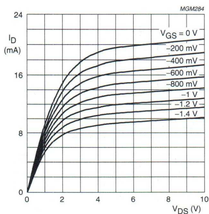
PMBFJ212.
