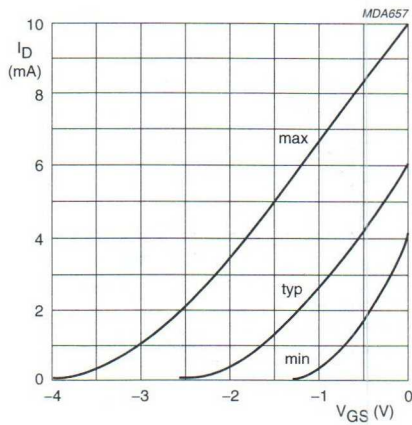
BFR30.
