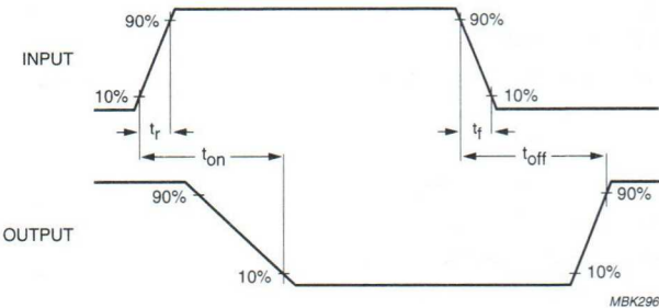
Fig.3 Switching times and input and output waveforms; R_i = 50\text{ }\Omega ; t_r < 0.5\text{ ns} ; t_f < 1.0\text{ ns} ; t_p = 20\text{ ns} ; \delta < 0.01 .
