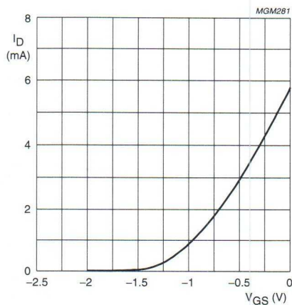
PMBFJ210.
