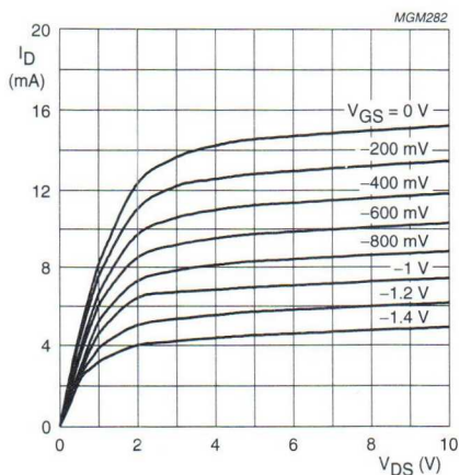
J211.
