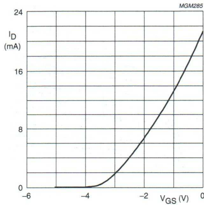
PMBFJ212.
