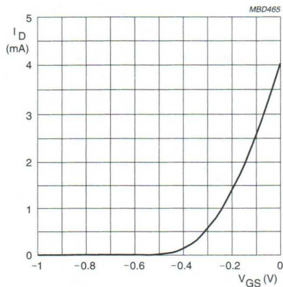
BF861A V_{DS} = 8 \text{ V.}
