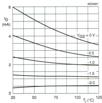
BFR30. V_{DS} = 10\text{ V}.
