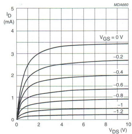
BFR31.
