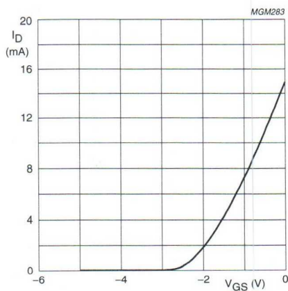
J211.
