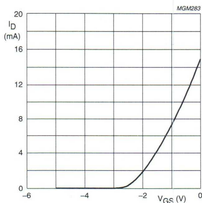
PMBFJ211.
