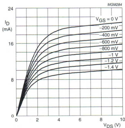
J212.
