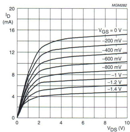
PMBFJ211.
