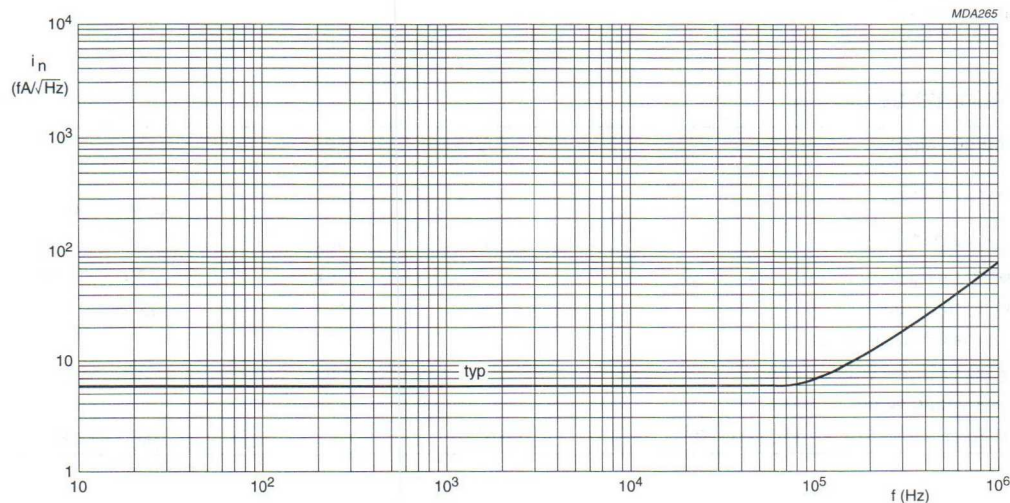
Fig.13 V_{DS} = 10 \text{ V} ; I_D = 0,2 \text{ mA} ; T_{amb} = 25 \text{ }^\circ\text{C} .
