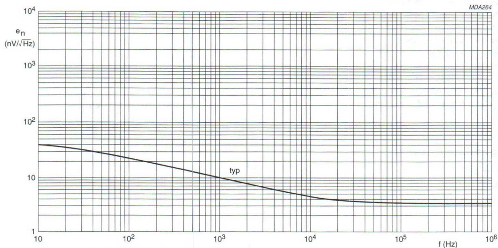
Fig.12 V_{DS} = 10 \text{ V} ; I_D = 0,2 \text{ mA} ; T_{amb} = 25 \text{ }^\circ\text{C} .
