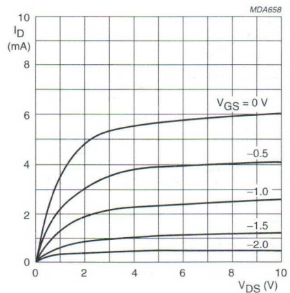
BFR30.
