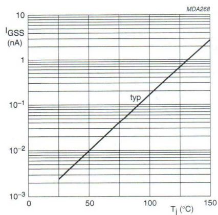
Fig.11 I_{GSS} versus T_j . -V_{GSS} = 10 V; V_{DS} = 0 .
