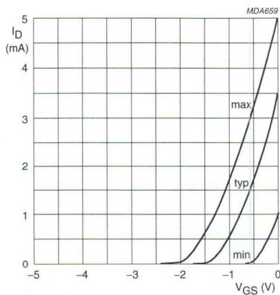
BFR31.
