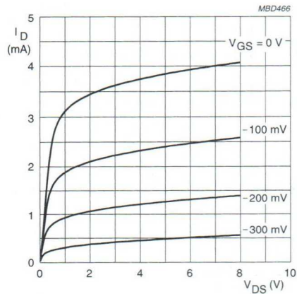
BF861A V_{DS} = 8 \text{ V.}
