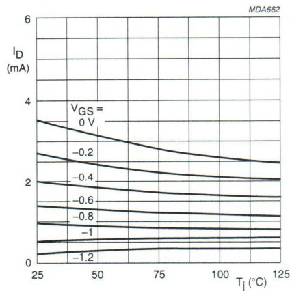
BFR31. V_{DS} = 10\text{ V}.
