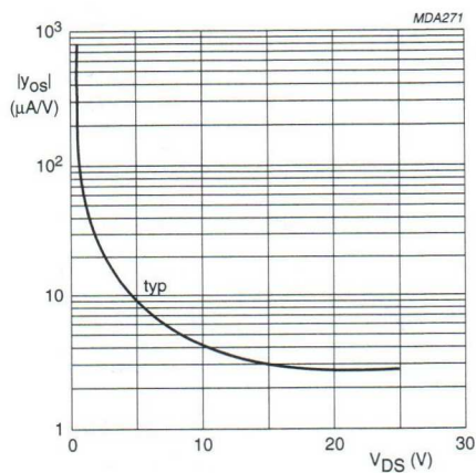
Fig.8 |y_{oss}| versus V_{DS} . I_D = 0,4 mA; f = 1 kHz; T_{amb} = 25 °C.
