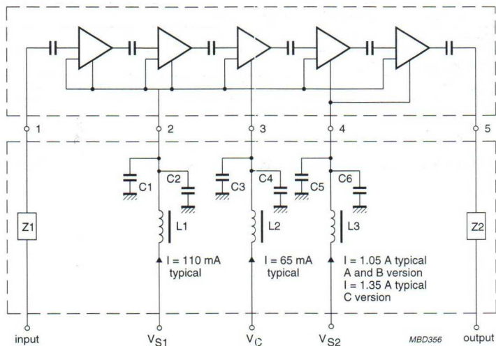
Fig.24 Test circuit.
