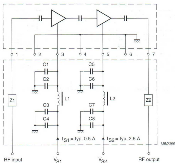
Fig.13 Test circuit.
