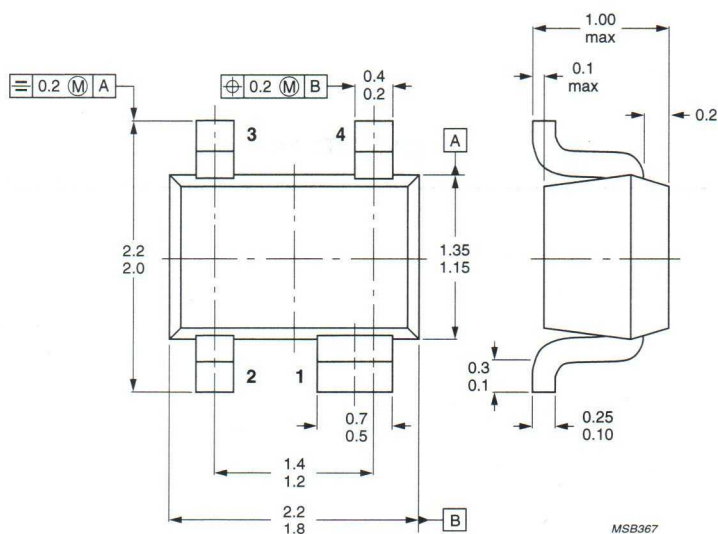
Fig.12 SOT343R.
