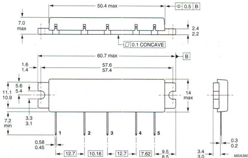
Fig.5 SOT278A.
