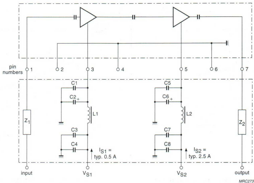
Fig.13 Test circuit.
