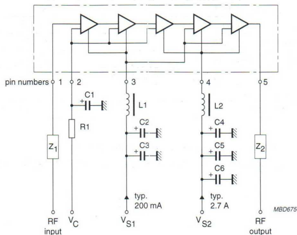
Fig.10 Test circuit.
