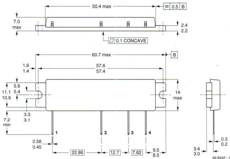
Fig.6 SOT278B.
