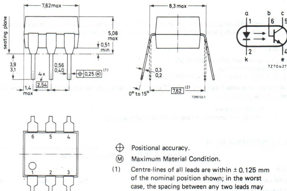
Fig.1 SOT90B.
