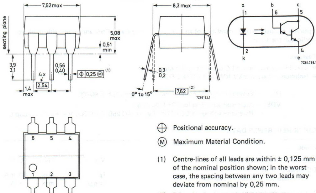
Fig.1 SOT90B.
