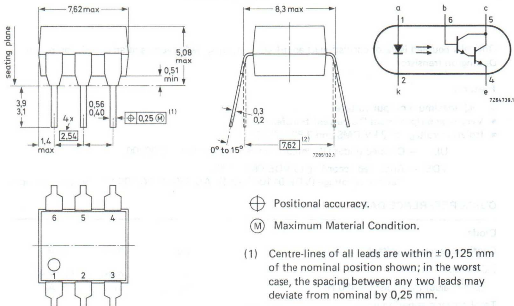
Fig. 1 SOT 90B.
