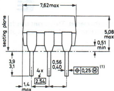
Fig.1 SOT90B.
