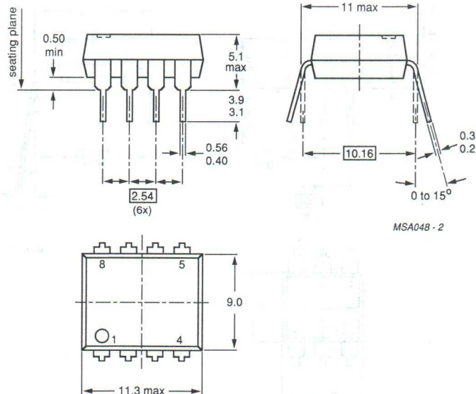
Fig.8 SOT271.
