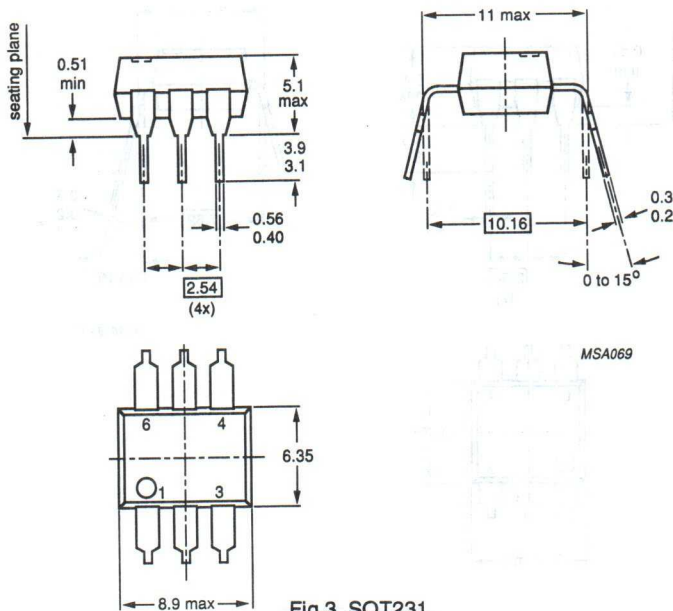
Fig.3 SOT231.
