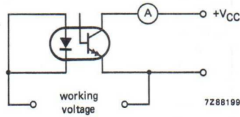
Fig. 2 Test circuit.
