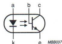
Fig.3 Symbol, CNX72A.
