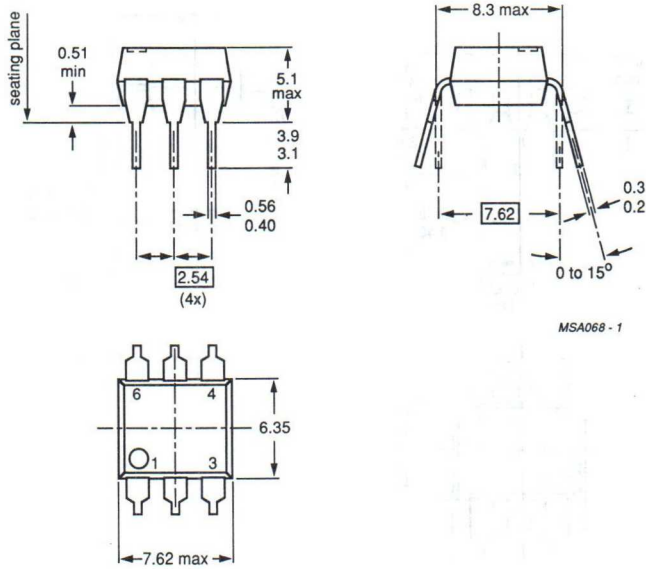
Fig.1 SOT90B.
