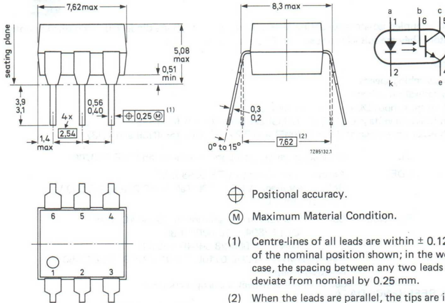
Fig. 1 SOT90B.
