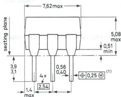
Fig. 1 SOT90B.
