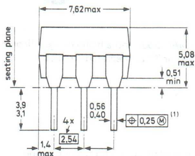
Fig.1 SOT90B.
