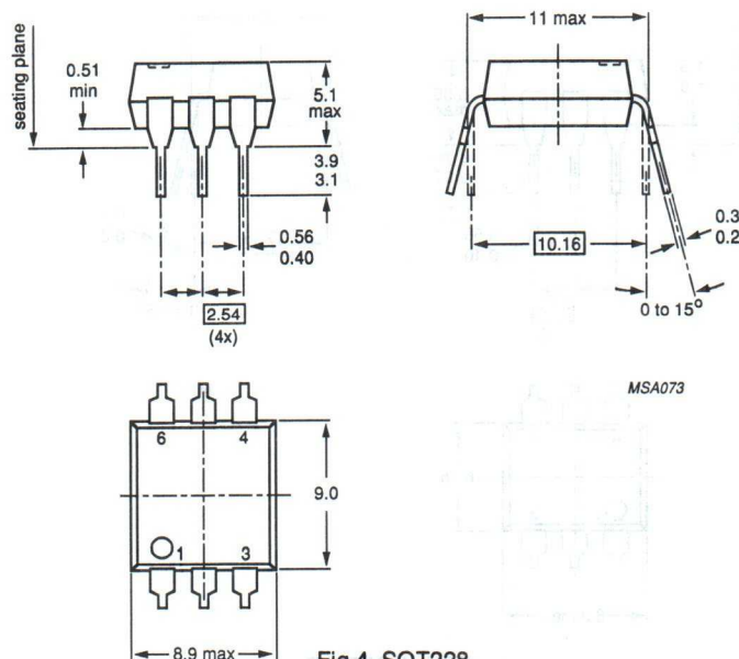
Fig.4 SOT228.
