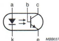
Fig.3 Symbol, CNX83A.
