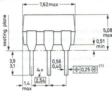
Fig.1 SOT90B.
