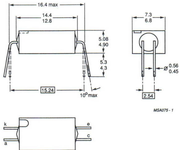
Fig.9 SOT211.
