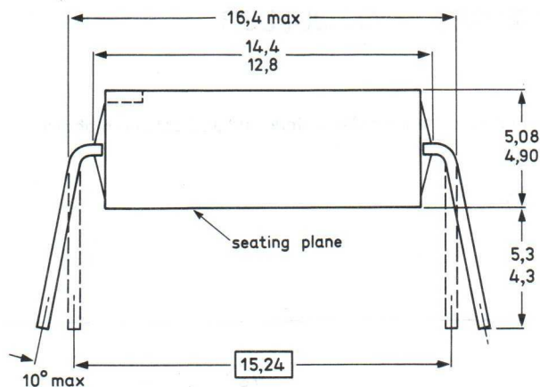
Fig. 1 SOT-211.
