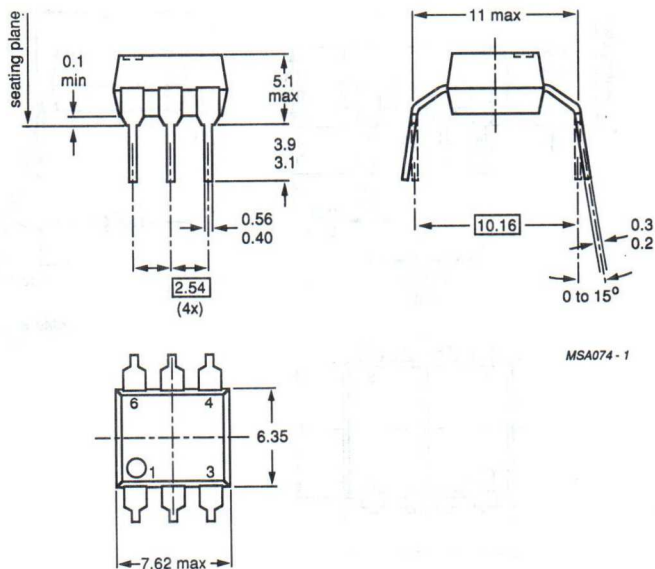
Fig.6 SOT212.
