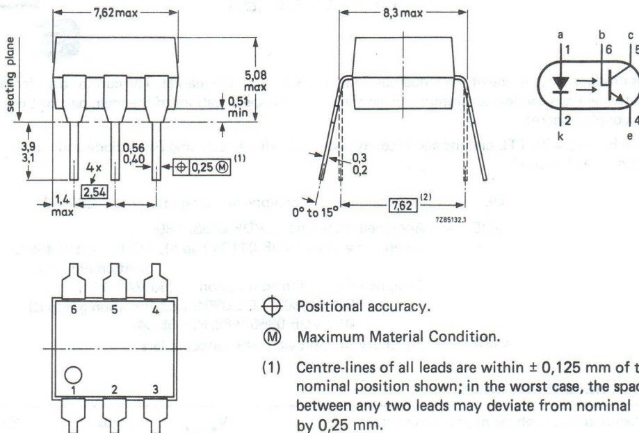
Fig. 1 SOT90B.
