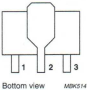
Fig.1 SOT89.
