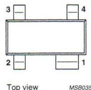
Fig.2 SOT143R.
