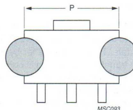
h. SOT223 ( P = 6.0 \text{ mm} ).
