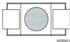
a. SOD106.
