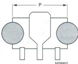
g. SOT89 ( P = 4.4 \text{ mm} ).
