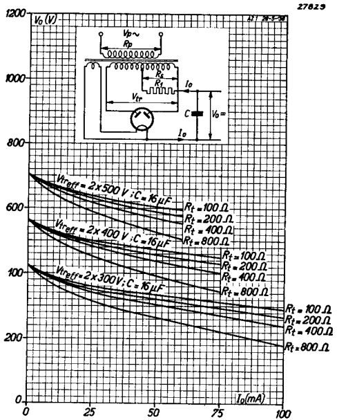
Abb. 4 Belastungskurven bei verschiedenen Transformatorerlaufspannungen und Innenwiderständen des Transformators ( R_t = R_s + u^2 R_p + R_l ).
