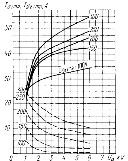
Усредненные импульсные характеристики: U_{g2} = 1 kV ; — анодные; - - - сеточно-анодные (по сетке второй) Averaged Peak Characteristic Curves: U_{g2} = 1 kV ; — anode; - - - grid 2-anode
