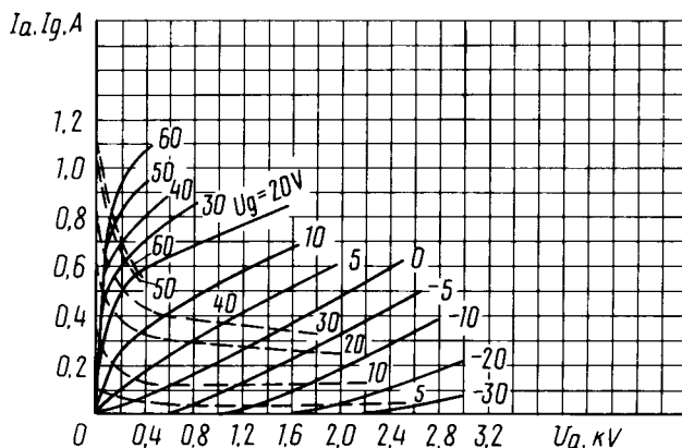
Усредненные анодные и сеточно-анодные характеристики: U_i = 12,6 В ————— анодные; - - - - - сеточно-анодные Averaged Anode and Grid-Anode Characteristic Curves: U_i = 12.6 V ————— anode; - - - - - grid-anode
