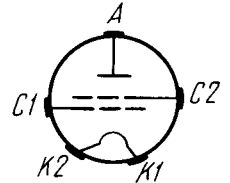
СХЕМА СОЕДИНЕНИЯ ЭЛЕКТРОДОВ С ВЫВОДАМИ CONNECTION OF ELECTRODES WITH LEADS
