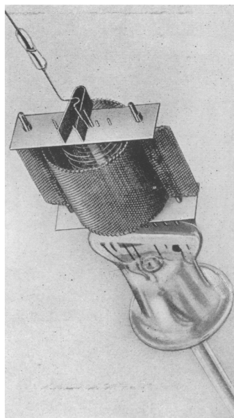
Innenkonstruktion der Endpenthode CL 1.
