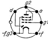
Sockelschaltenschema
