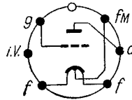
Sockelschaltschema
