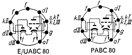
Sockelschaltenschema
