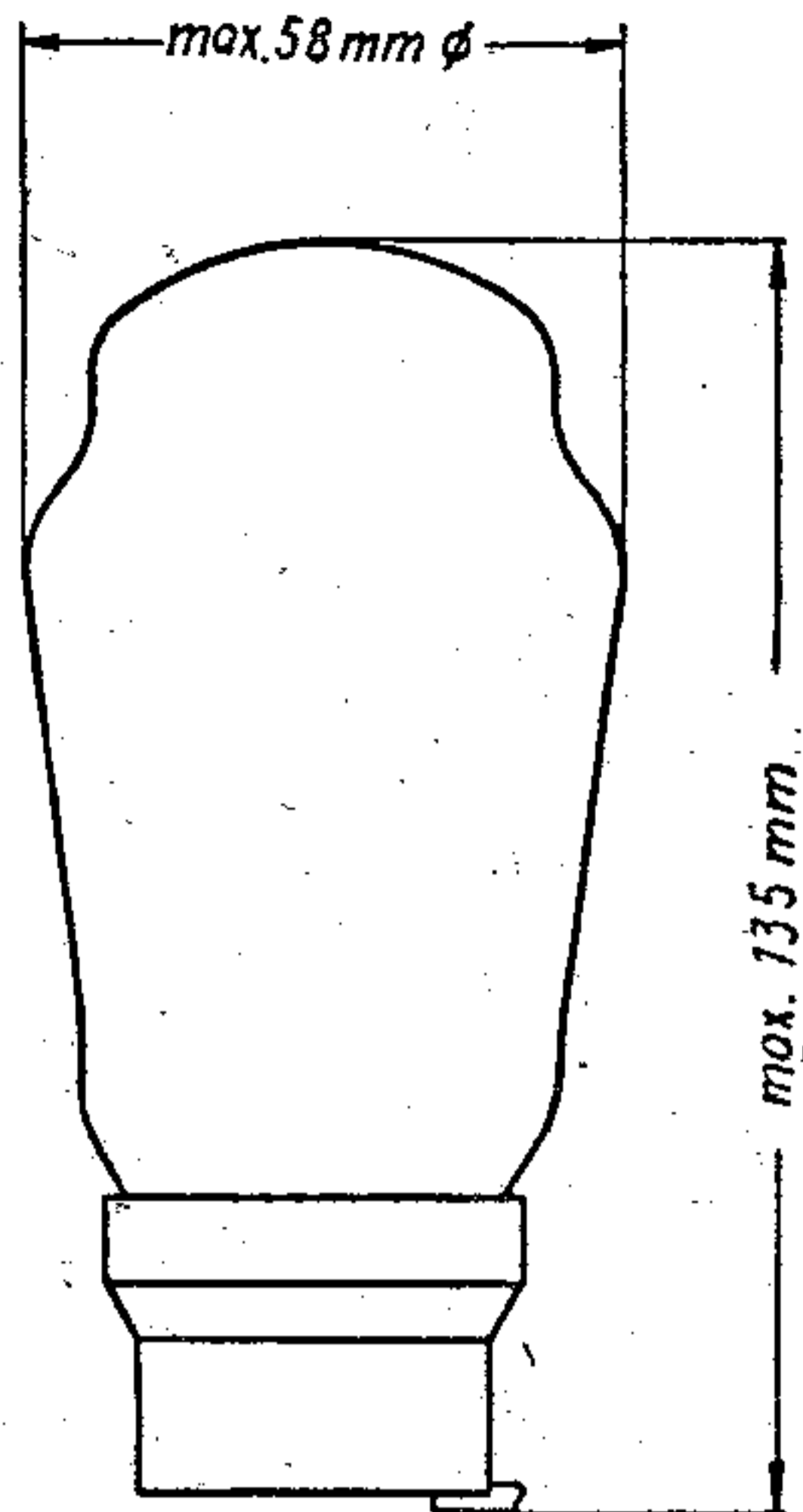
Kolbengröße
