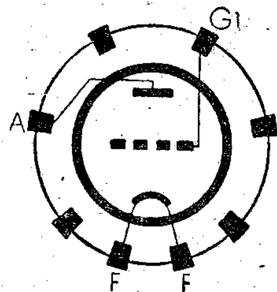
Sockelschaltung
