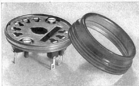
Bild 108. Stahlröhrenfassung mit Gewindering und Überwurfmutter zur Verwendung für ECF 12/UCF 12
