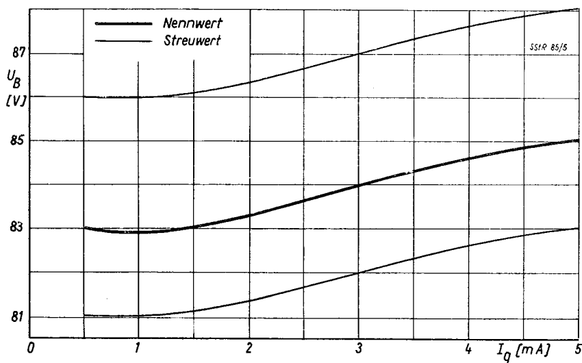
Brennspannungskennlinie
