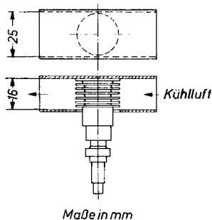
Kühlluft-Leitstück
